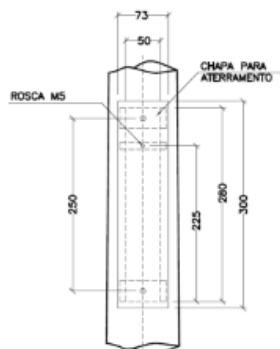
DETALHE C
